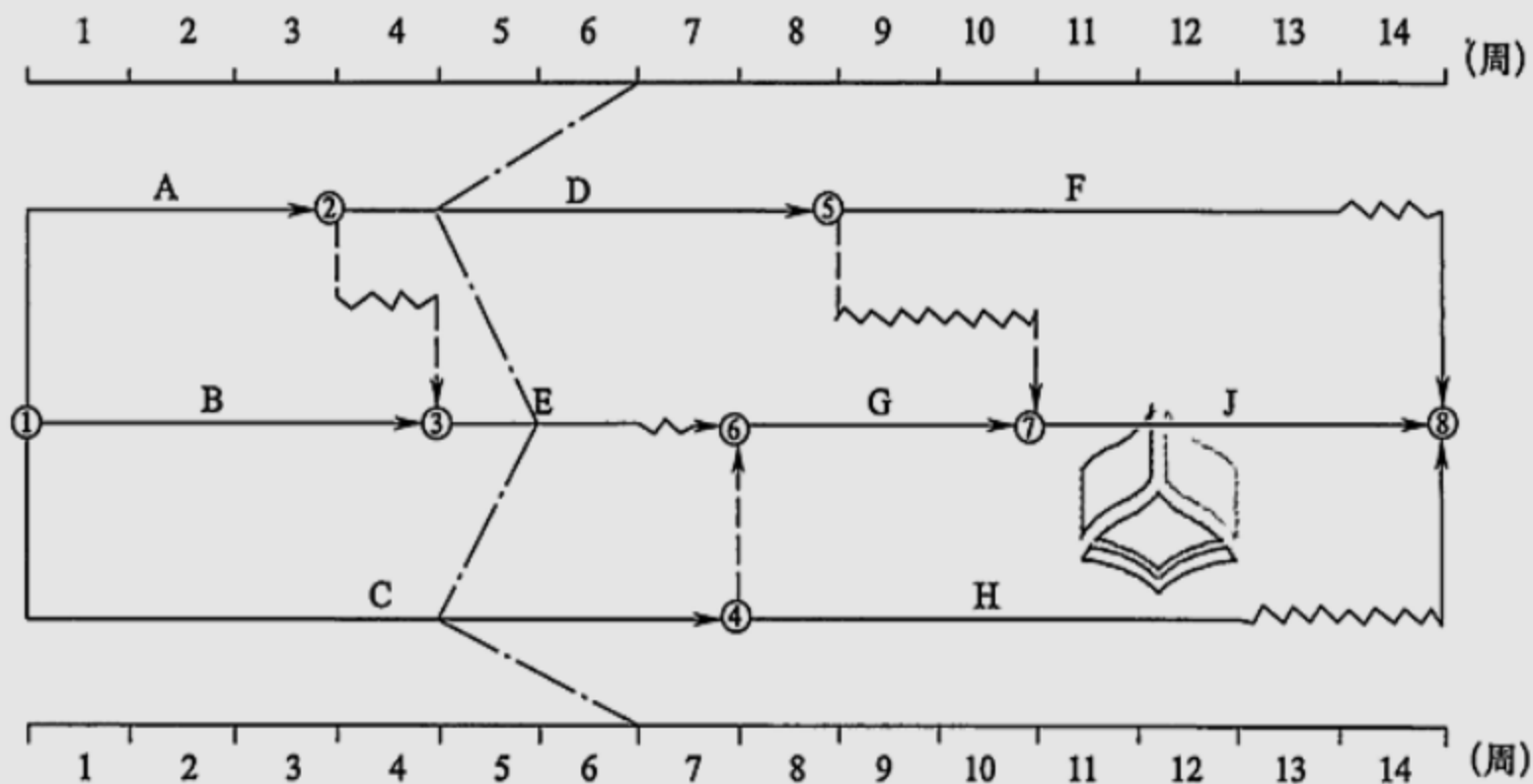
图 5-13 某工程实际进度前锋线比较
