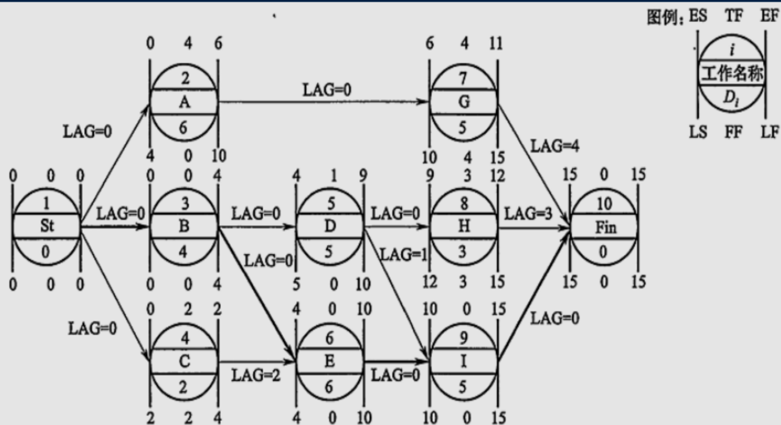
图 5-9 单代号网络计划
