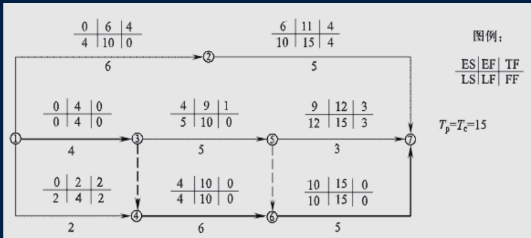
图5-3双代号网络计划（六时标注法）
