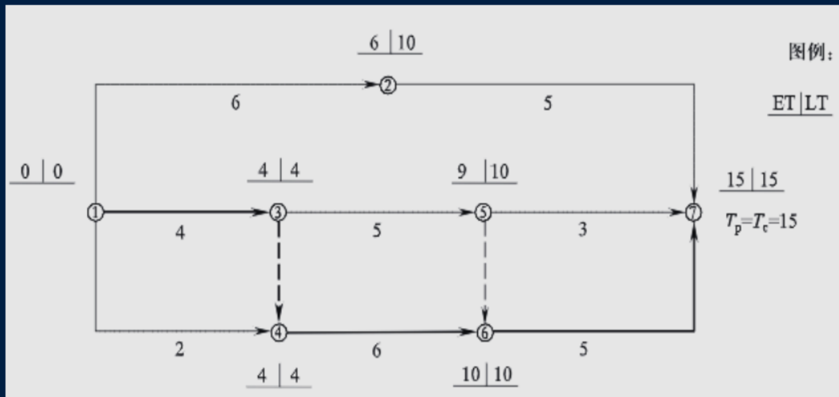
图5-5双代号网络计划（按节点计算法）
