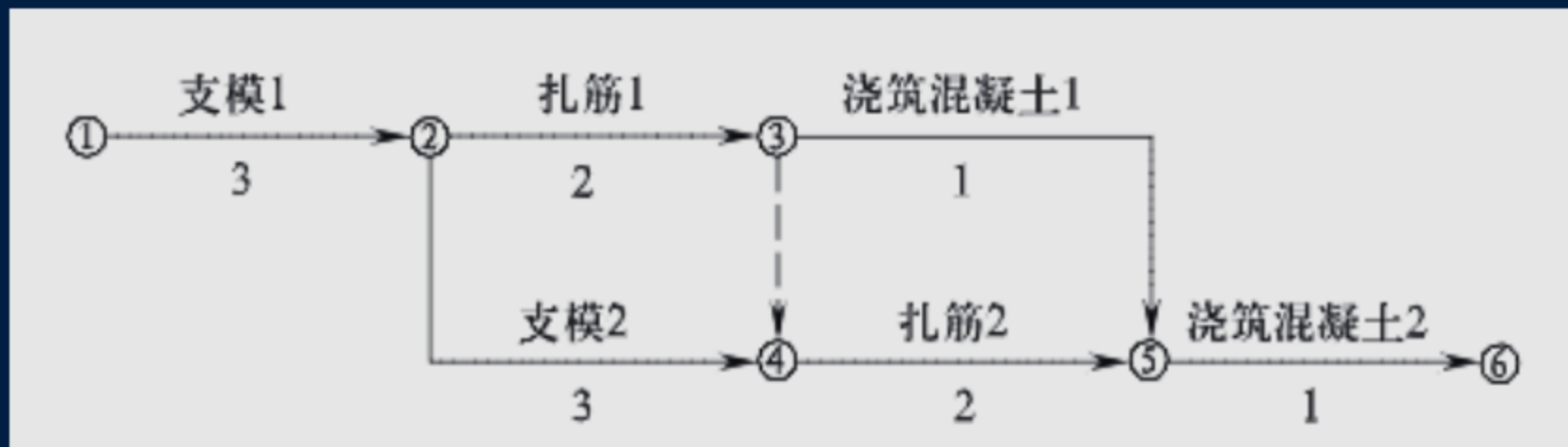
图5-1某混凝土工程双代号网络计划
