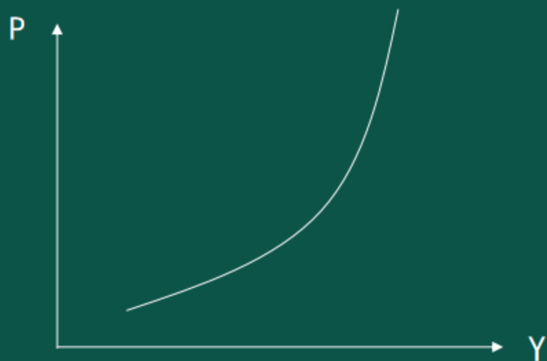
短期总供给曲线
